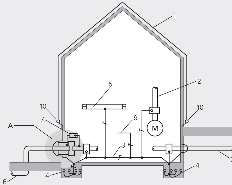
4.4.3 Figure 2: Disposition d'un éclateur et des liaisons équipotentielles de protection
