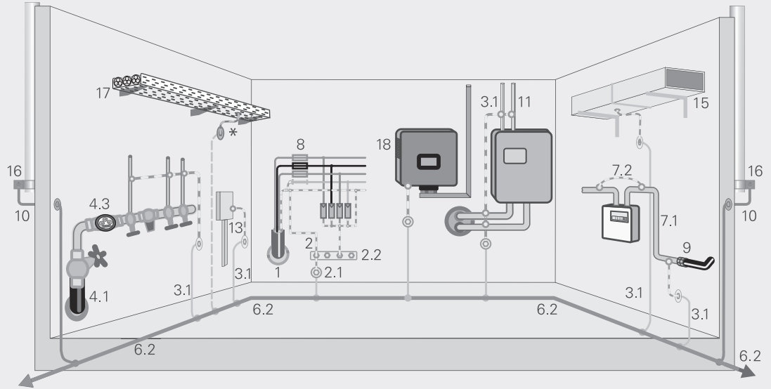
4.1.1 Figure 1: Liaison équipotentielle de protection
