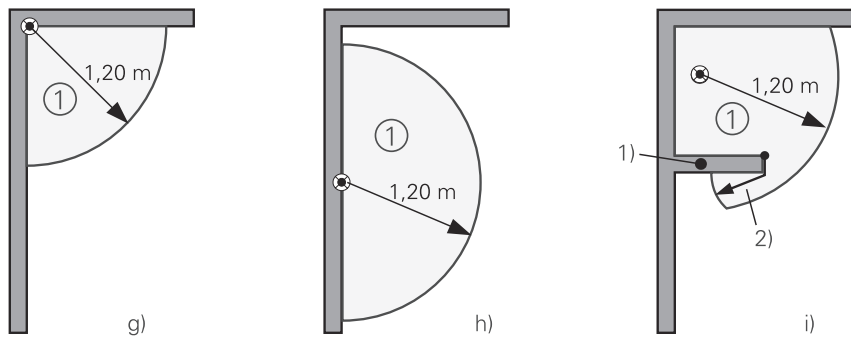
7.01.3 Figure 3: Douches sans receveur dans les vestiaires d'installations sportives etc.: dimensions du volume 1
