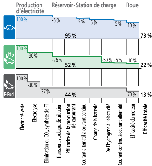
Figure 5.4: Tank-to-Wheel «Véhicule électrique H2 contre E-Fuel»
