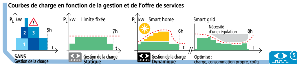
Figure 13.5: Courbes de charge en fonction de la gestion et de l'offre de services
