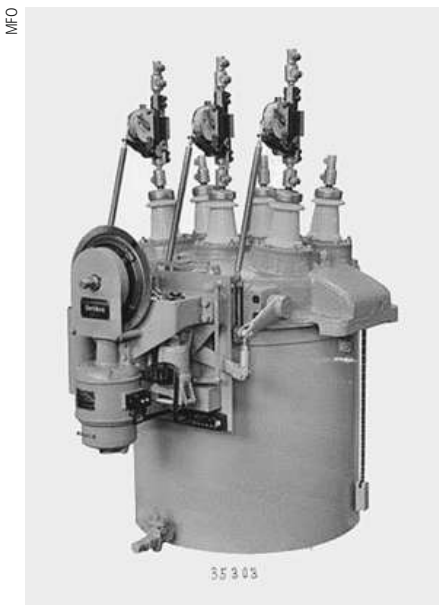
Bild 1 Ölkeschalter mit Primärauslöser HZM, MFO, 1912, BBC.
