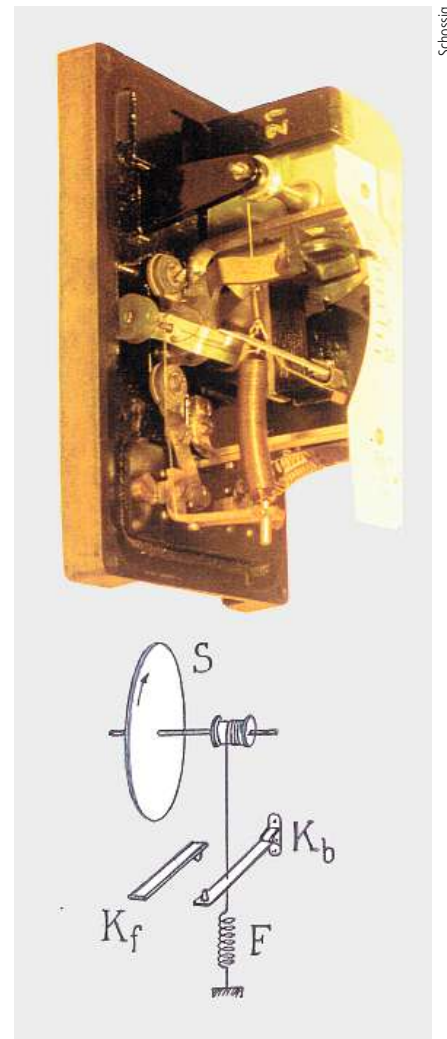
Bild 2 Überstromrelais RA1, S&H, 1925.
