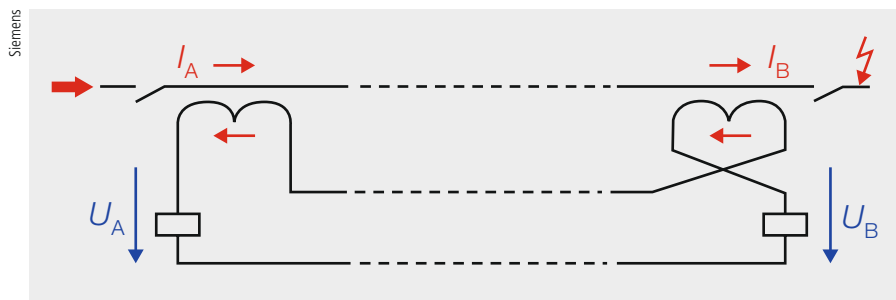
Bild 3 Differenzialschutz nach Merz und Price mit gegeneinander geschalteten Wandlern.
